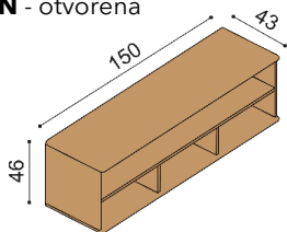
Komoda FLABO FL3PN - otvorená
