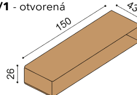
Komoda FLABO FL3/1 - otvorená
